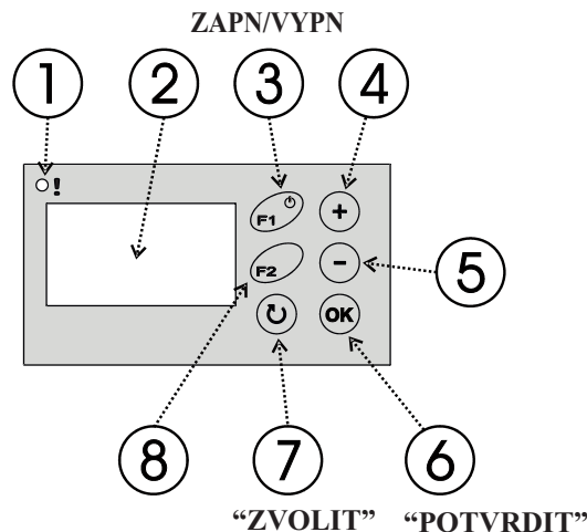
Obr. 2 Ovládací panel
